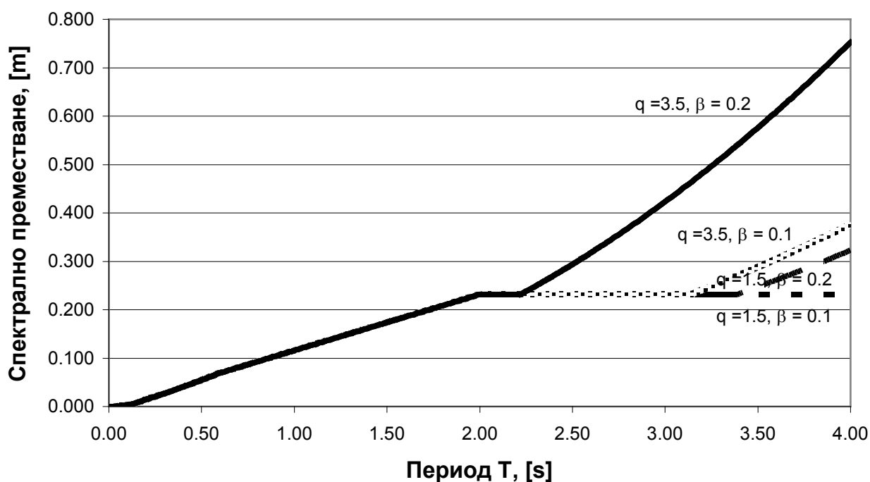
Фигура NA.4.8.6 - Изчислителен спектър на преместванията за почва тип С
