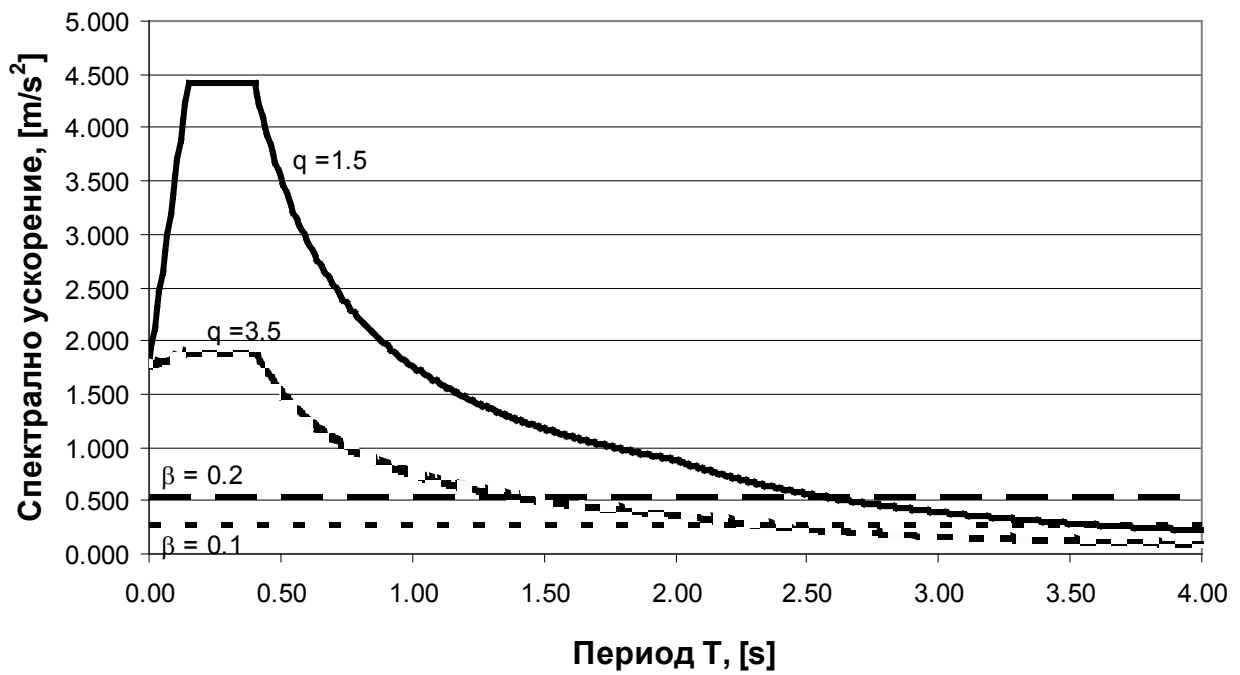
Фигура NA.4.8.1 - Изчислителен спектър на ускоренията за почва тип А
