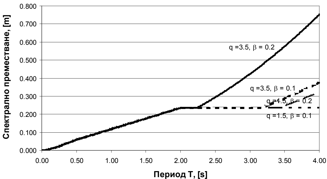
Фигура NA.4.8.10 - Изчислителен спектър на преместванията за почва тип E.
