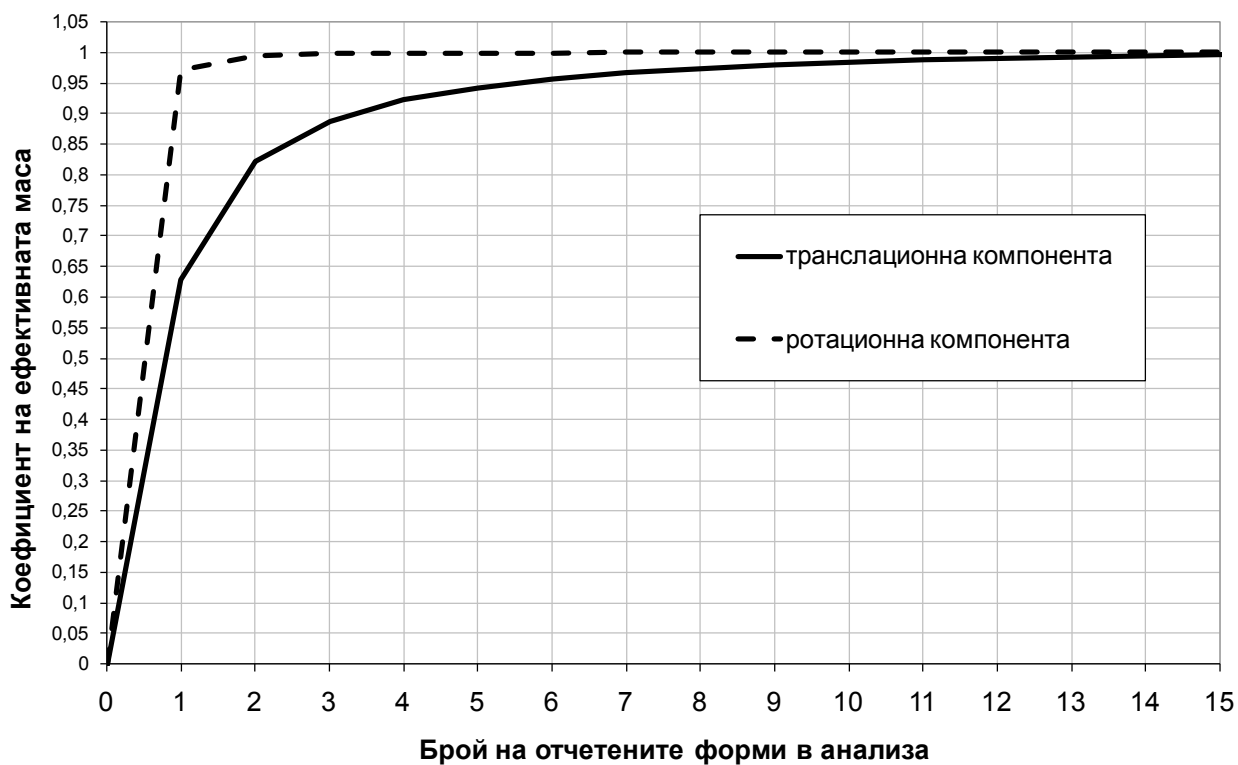
Фигура NA.4.4.5 - Коефициент на ефективната маса в зависимост от броя на включените в анализа форми: плътна линия – изследване за транслационната компонента; прекъсната линия – изследване за ротационната компонента
