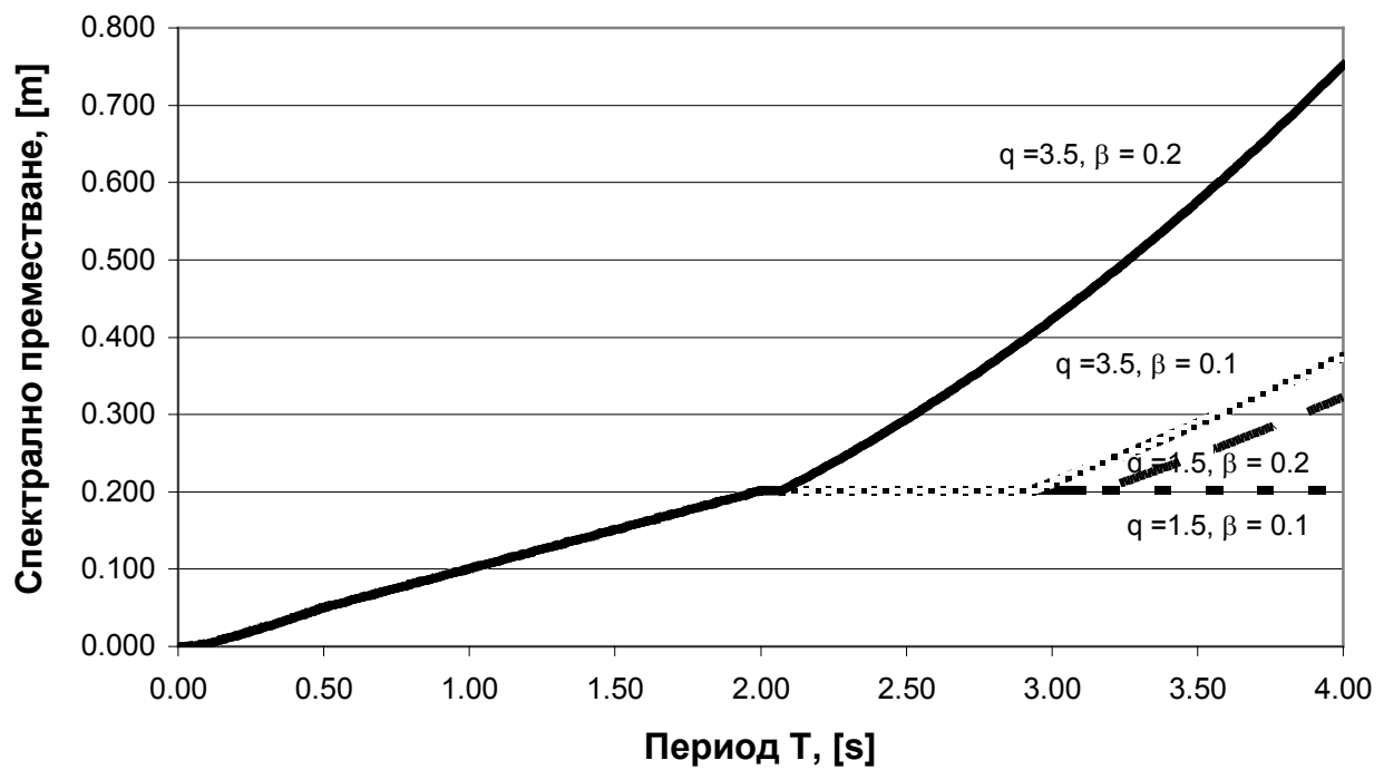
Фигура NA.4.8.4 - Изчислителен спектър на преместванията за почва тип В
