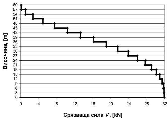
Фигура NA.4.10.2 - Разпределение на срязващите сили по височина при форма 1
