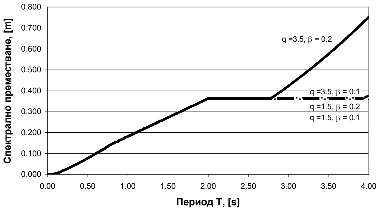
Фигура NA.4.8.8 - Изчислителен спектър на преместванията за почва тип D
