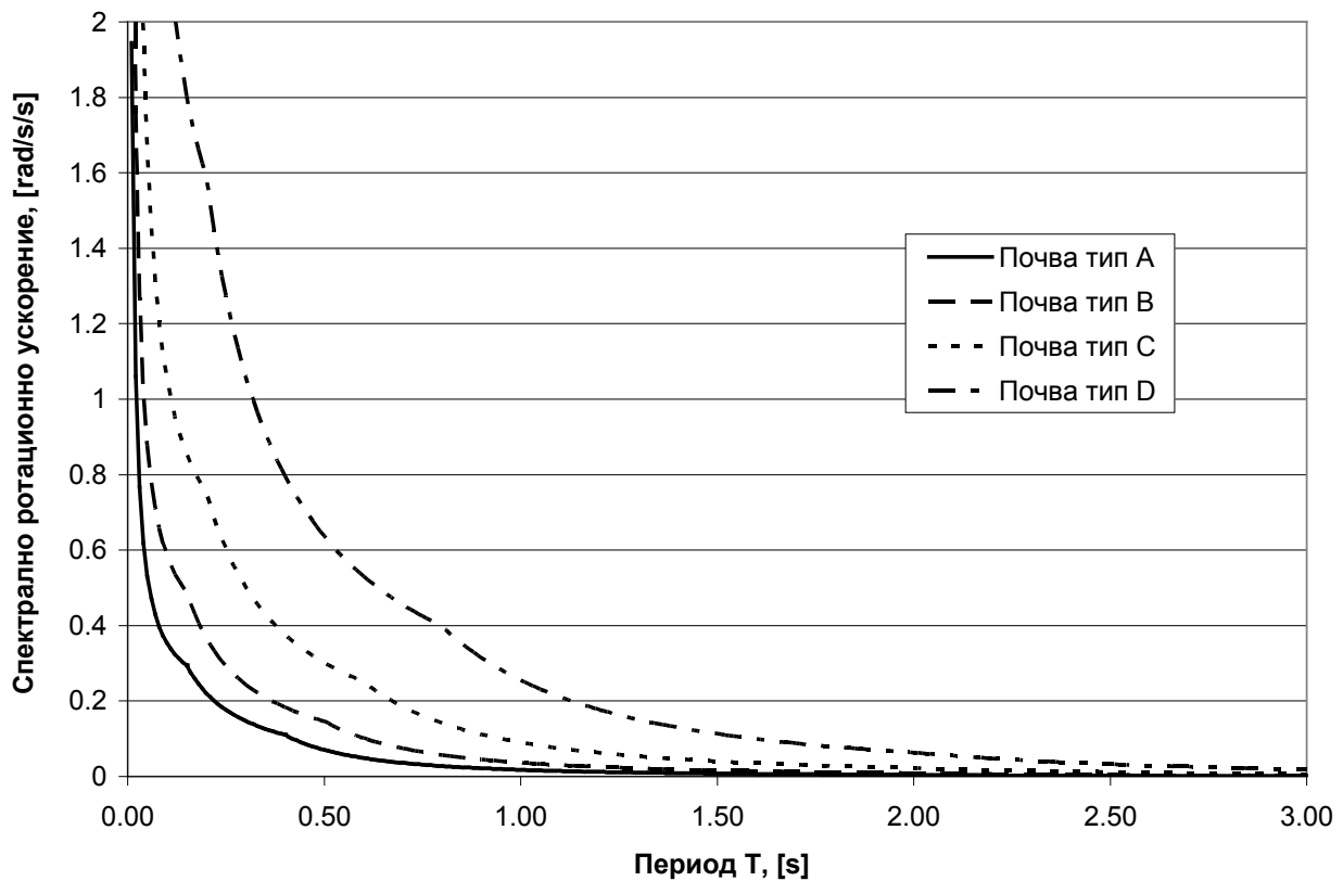
Фигура NA.4.1.2 - Еластичен спектър на реагиране за ротационната компонента около хоризонтална ос (за типове почви А, В, С и D), скалирани за изчислително ускорение 0,27g
