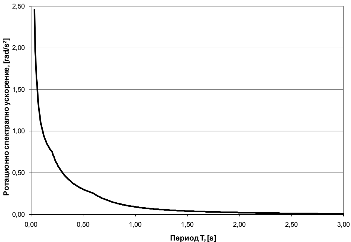
Фигура NA.4.4.4 - Еластичен спектър на ротационните ускорения за почва тип С според БДС EN1998-1:2004, скалиран към изчислително почвено ускорение 0,27g и затихване 5%
