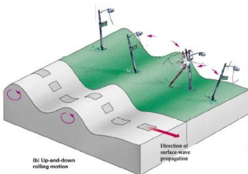
Фигура NA.4.1.4 - Илюстрация на влиянието на ротационната компонента върху корави стълбове (малък фундаментален период)
