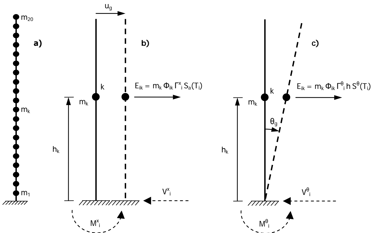
Фигура NA.4.1.5 - Стотанена кула с височина 60 m, дискретизирана с 20 елемента и 21 възли (тръбно сечение с диаметър 1,20 m и дебелина на стената 0,03 m): а) дискретен модел; б) случай на транслационно преносно движение; в) случай на ротационно преносно движение
