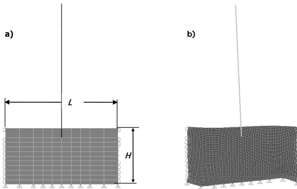
Фигура NA.4.3.3 - Модел на почва – конструкция: а) геометрия, размери и подпиране на земния масив; б) симулиране на ротационна компонента чрез вълново синусоидално движение на скалния пласт.
