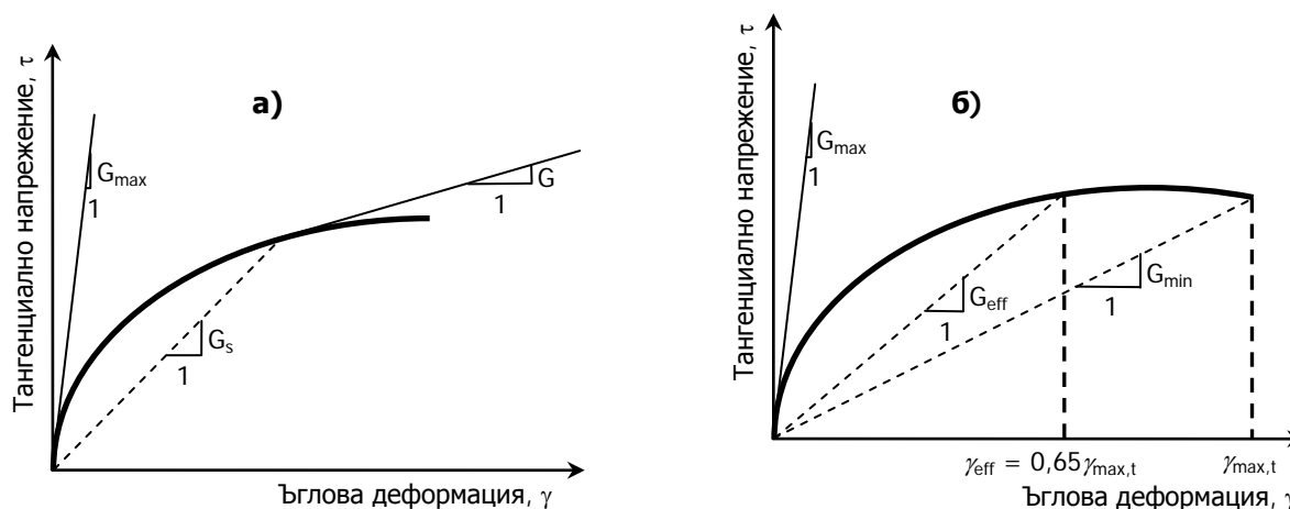
Фигура NA.4.3.4 - Зависимост тангенциално напрежение – ъглова деформация: а) модул на ъгловите деформации – начална стойност G_{max} , секуща стойност G_s и тангенциална стойност G ; б) определяне на ефективните стойности G_{eff} и \gamma_{eff} ; G_{min} и \gamma_{max,t} .
