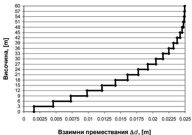
Фигура NA.4.10.3 - Разпределение на взаимните премествания по височина при форма 1
