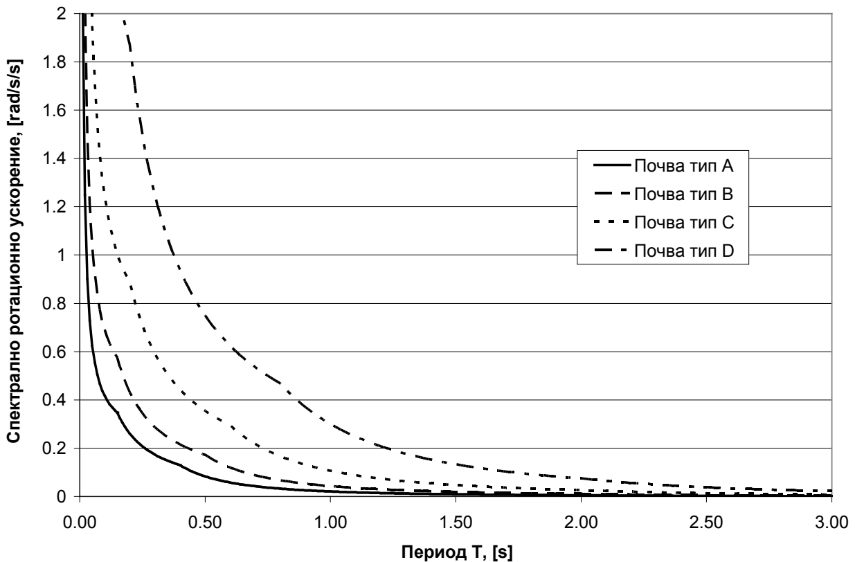
Фигура NA.4.1.3 - Еластичен спектър на реагиране за ротационната компонента около вертикална ос (за типове почви А, В, С и D), скалирани за изчислително ускорение 0,27g
