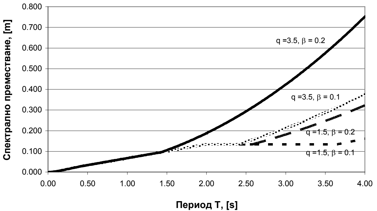
Фигура NA.4.8.2 - Изчислителен спектър на преместванията за почва тип А
