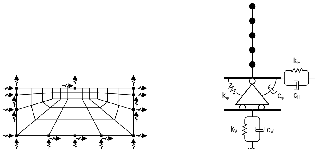
Фигура NA.4.3.2 - Приблизителен анализ на конструкцията чрез разделяне на почвения масив и конструкцията над него
