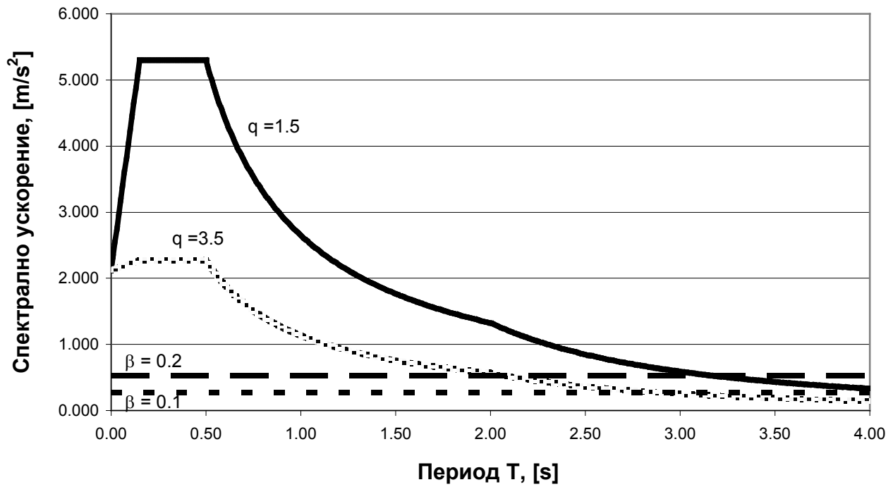
Фигура NA.4.8.3 - Изчислителен спектър на ускоренията за почва тип В
