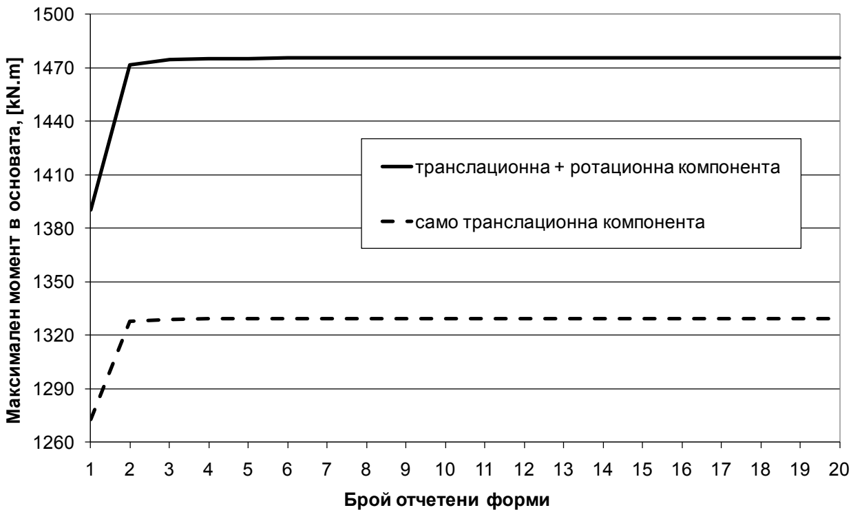
Фигура NA.4.4.7 - Зависимост на максималния момент в основата на кулата от броя на включените в анализа форми: прекъсната линия – отчетена е само транслационната компонента на сеизмичното въздействие; плътна линия – отчетени са транслационната и ротационната компоненти на сеизмичното въздействие
