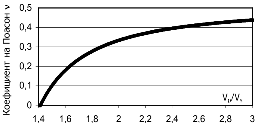
Фигура NA.4.3.5 - Определяне на ефективната стойност на коефициента на Poisson \nu в зависимост от отношението на скоростите на надлъжната ( V_p ) и напречната ( V_s ) вълни
