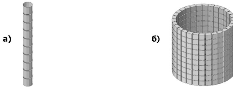
Фигура NA.4.4.1 - а) Конзолен модел с прътови крайни елементи; б) пространствен модел с черупкови крайни елементи.
