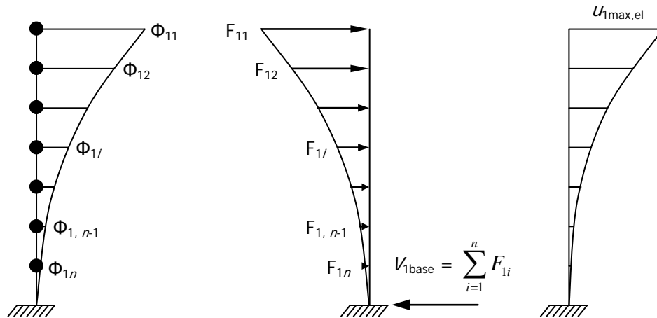
Фигура НА.4.10.1 - Последователност на стъпките за реализиране на метода на хоризонталното натоварване
