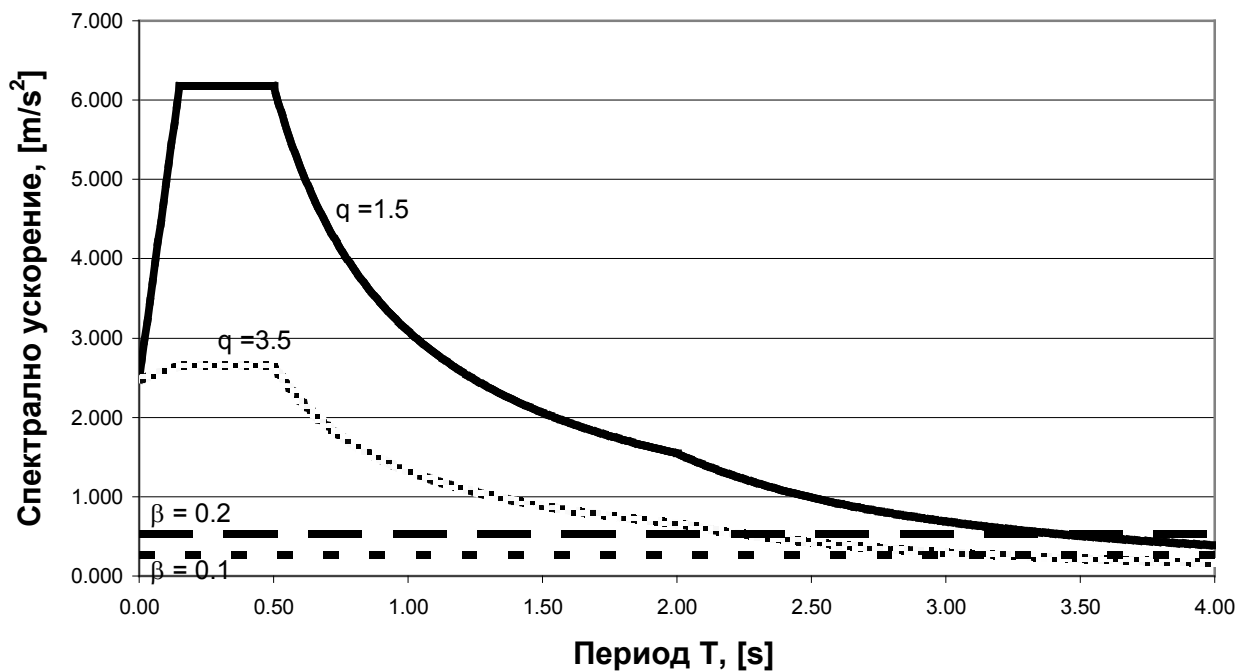
Фигура NA.4.8.9 - Изчислителен спектър на ускоренията за почва тип E
