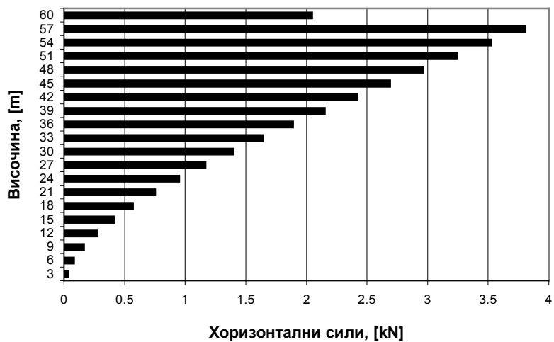
Фигура NA.4.10.4 - Разпределение на хоризонталните сили по височина при форма 1
