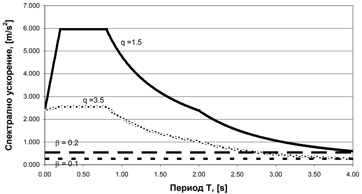
Фигура NA.4.8.7 - Изчислителен спектър на ускоренията за почва тип D
