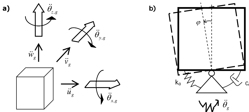
Фигура NA.4.1.1 - а) Шест компоненти на сеизмичното въздействие (ускорение) в основата – три транслационни и три ротационни; б) система с една степен на свобода при ротационно движение на масата.
