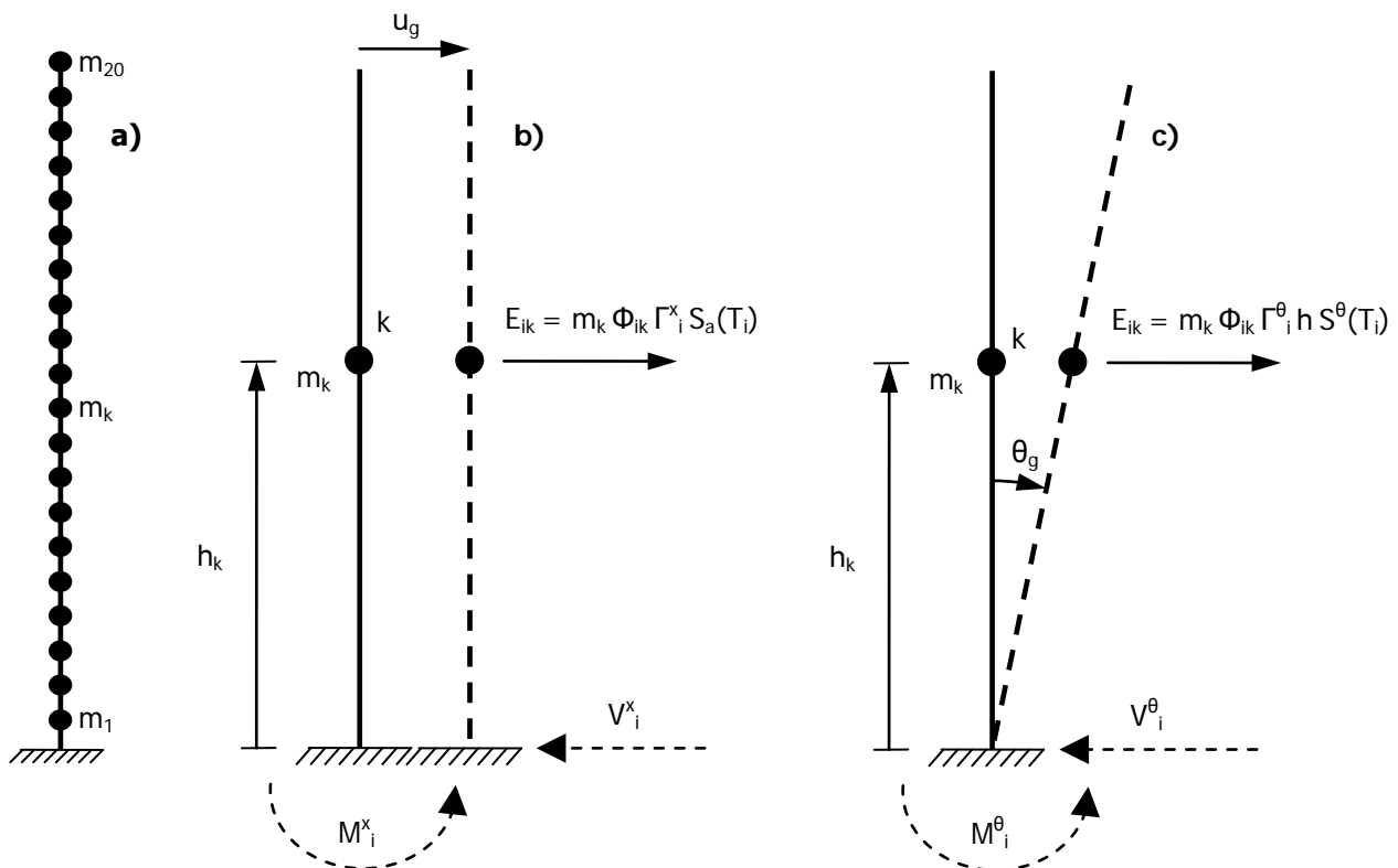
Фигура NA.4.4.2 - Стоманена кула с височина 60 m, дискретизирана с 20 елемента и 21 възли (тръбно сечение с диаметър 1,20 m и дебелина на стената 0,03 m): а) дискретен модел; б) случай на транслационно преносно движение; в) случай на ротационно преносно движение.
