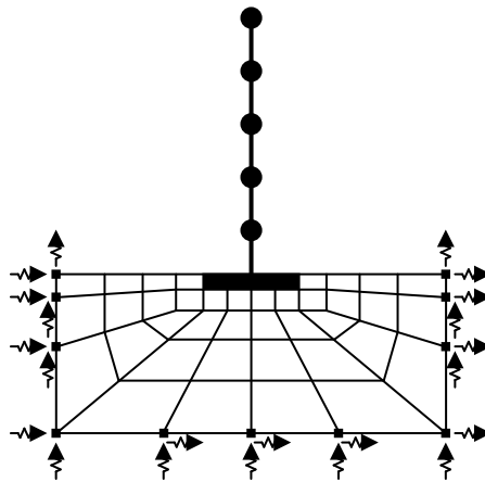
Фигура NA.4.3.1 - Изчислителен модел по метода на крайните елементи за отчитане на взаимодействието почва – конструкция.
