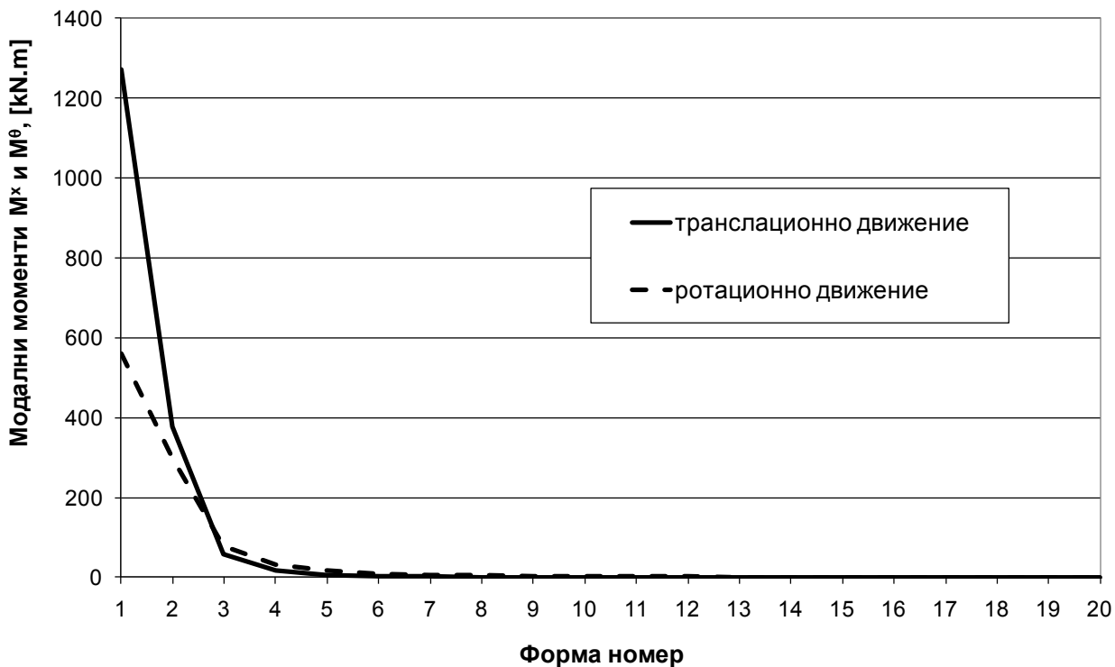
Фигура NA.4.4.6 - Модален огъващ момент в основата на кулата (за всяка от двайсетте форми): плътна линия – при действие само на транслационната компонента на ускоренията в основата; прекъсната линия – при действие само на ротационната компонента на ускоренията в основата
