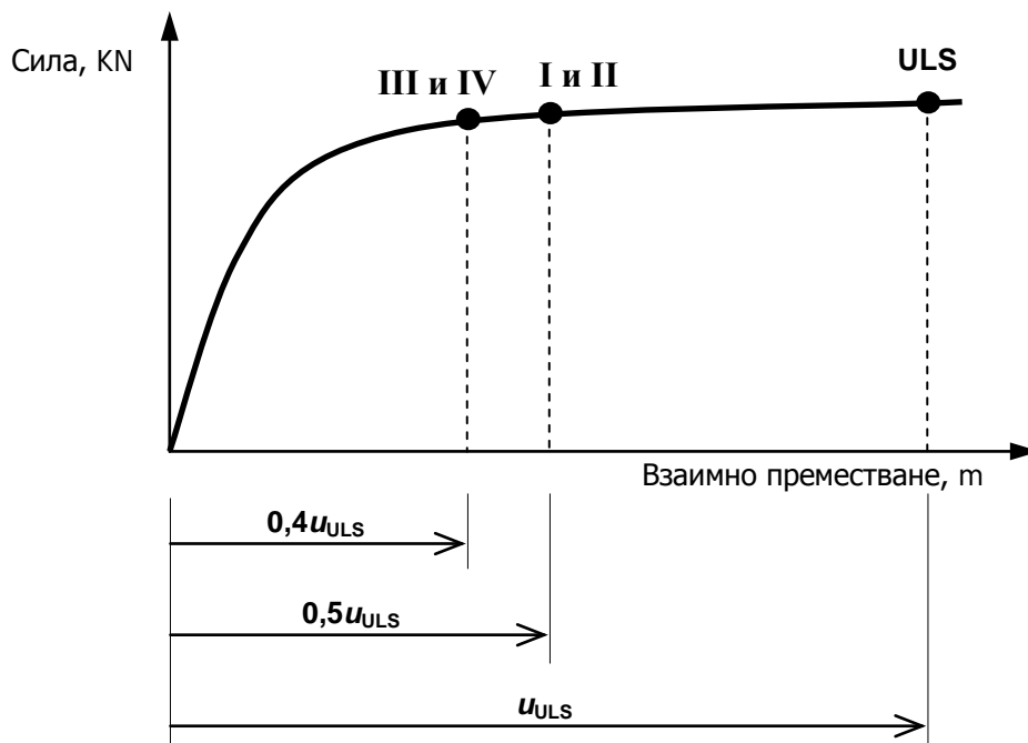
Фигура NA.4.12.1 - Към обяснението за избор на коефициентите \nu за определяне на граничното състояние на ограничени повреди за конструкции с различни класове на значимост
