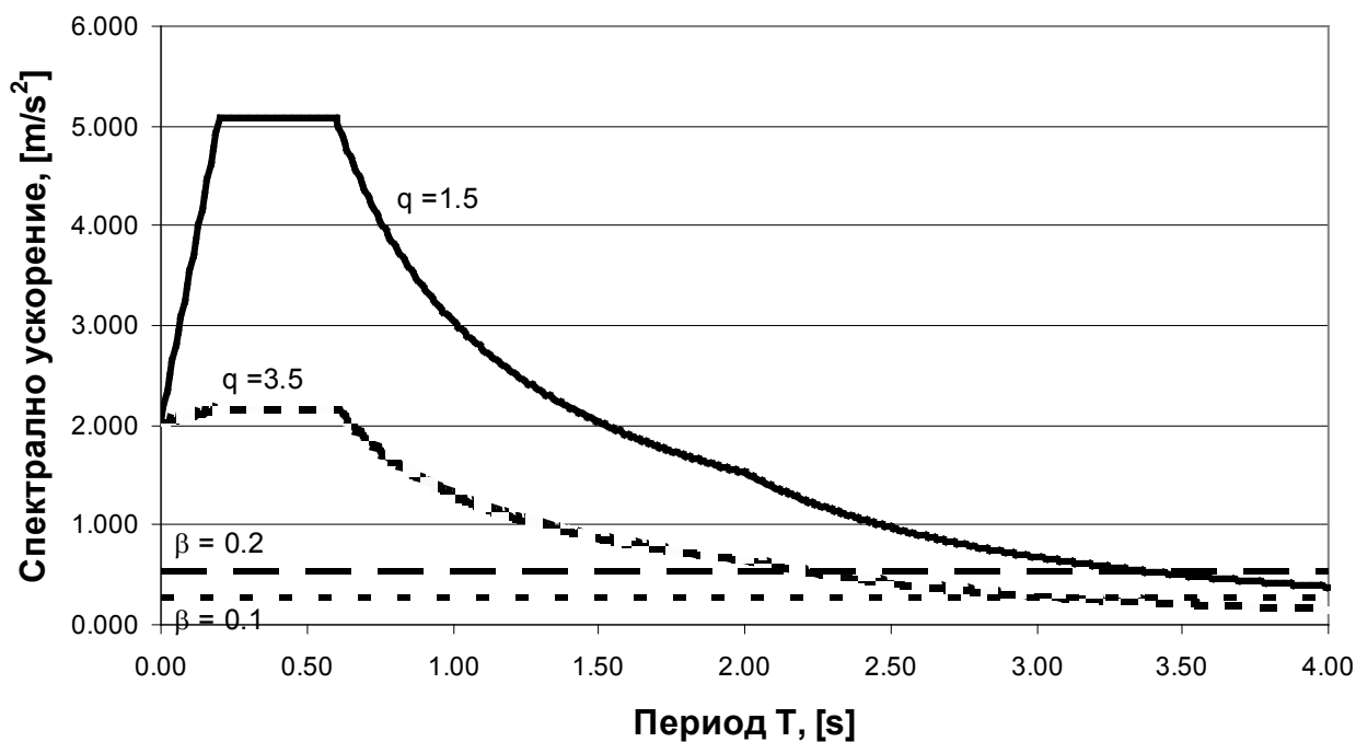
Фигура NA.4.8.5 - Изчислителен спектър на ускоренията за почва тип С.
