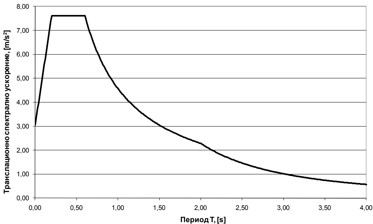
Фигура НА.4.4.3 - Еластичен спектър на транслационните ускорения за почва тип С според БДС EN1998-1:2004, скалиран към изчислително почвено ускорение 0,27g и затихване 5%
